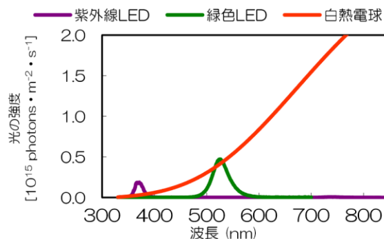
図Ⅶ-7-3 LED と白熱電球のスペクトル
