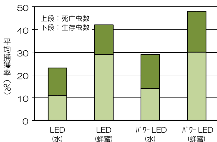
図Ⅶ-14-8 試作した LED 採集装置によるギフアブラバチの誘引効果
